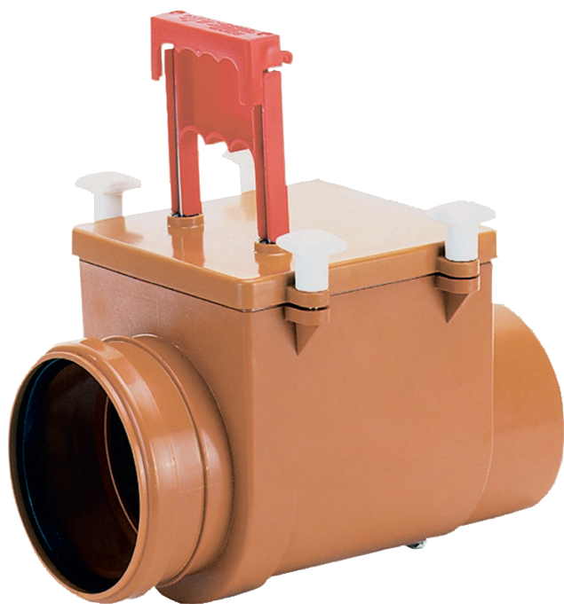
HL710.1 Механический канализационный затвор
